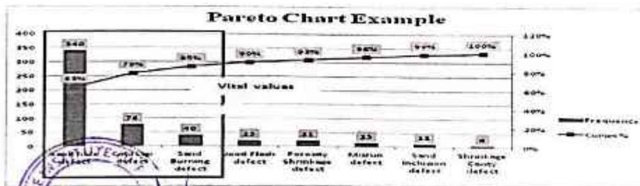
Fig. 6 Pareto charts
